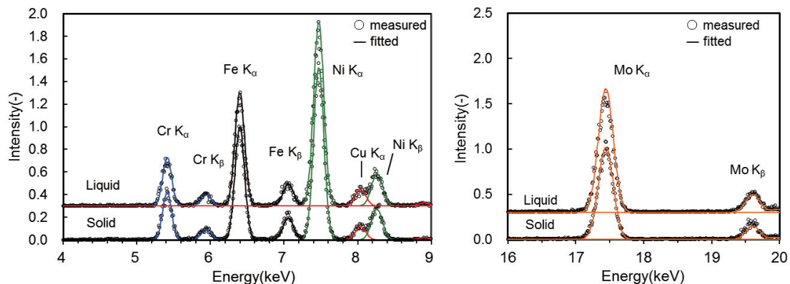
図 3. 固液界面近傍の固相および液相の蛍光 X 線スペクトルの測定例 (Fe-23Cr-40Ni-3Mo-2Cu 合金)
