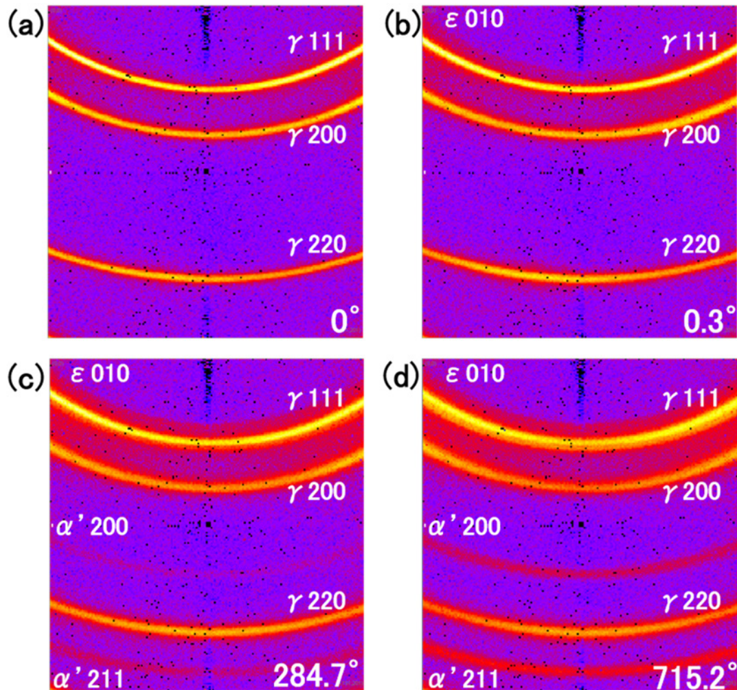
図 1 ねじり変形の進行に伴う回折パターン変化 (a) ねじり角 0°、(b) ねじり角 0.3°、(c) ねじり角 284.7°、(d) ねじり角 715.2°
